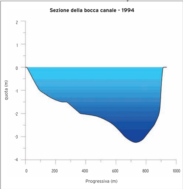
Figura 21: profilo batimetrico della bocca lagunare nel 1994 (visuale verso mare); la linea rossa sul DEM indica l'ubicazione della sezione. Sfondo: Volo ReVen 1990.
