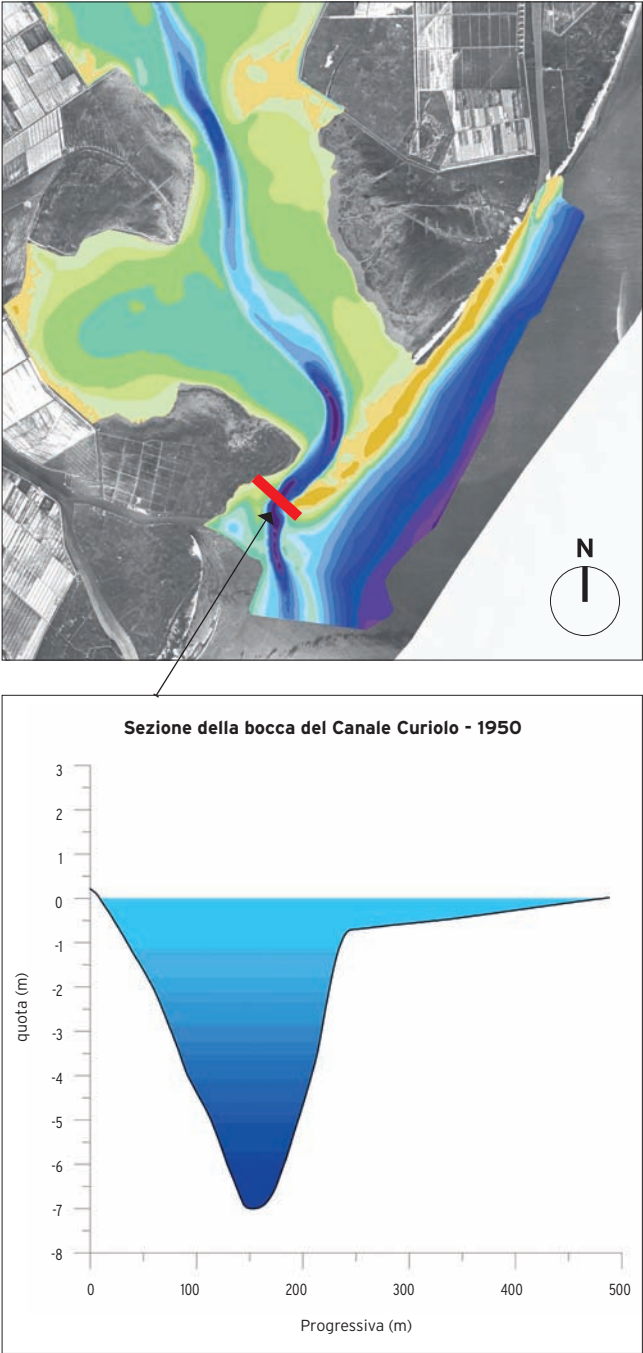
Figura 19: profilo batimetrico della bocca lagunare nel 1950 (visuale verso mare); la linea rossa sul DEM indica l'ubicazione della sezione. Sfondo: Voilo GAI 1955.
